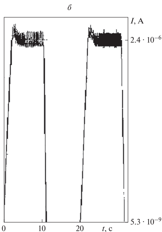
Рис. 1. Изменение тока пленки LiF/Cu, соответствующее краткосрочной памяти, при подаче импульсов напряжения через интервал времени 2 с (а) и соответствующее долгосрочной памяти при периоде импульсов напряжения 20 с (б).
